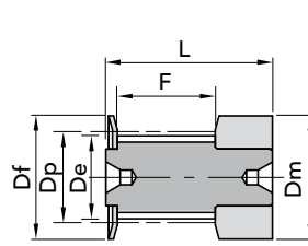
ESEC. 0F
