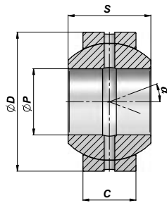
TYPE FO
