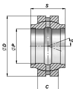
TYPE LO
