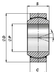
TYPE UK...2RS
